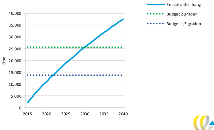
Figuur 7 - Cumulatieve CO 2 -uitstoot van Den Haag bij gemeentelijk en landelijk vastgesteld en voorgenomen beleid
